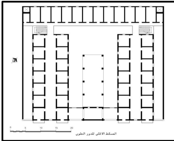
شكل رقم (٢) مسقط أفقي يوضح تخطيط الطابق العلوي لبازار الخديوي عباس بمدينة بورسعيد عمل الباحث
