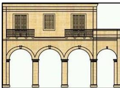
شكل رقم (٤) قطاع رأسى يوضح تفاصيل القسم الأيسر من الواجهة الرئيسية الجنوبية الشرقية للبازار - عمل الباحث
