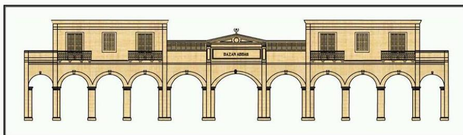
شكل رقم (٣) قطاع رأسى يوضح تفاصيل الواجهة الرئيسية الجنوبية الشرقية لبازار الخديوى عباس عمل الباحث
