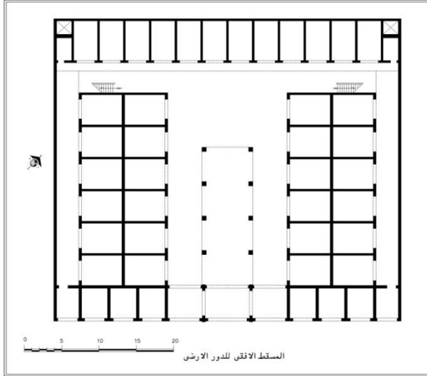
شكل رقم (١) مسقط أفقي يوضح تخطيط الطابق الأرضي لبازار الخديوي عباس بمدينة بورسعيد عمل الباحث
