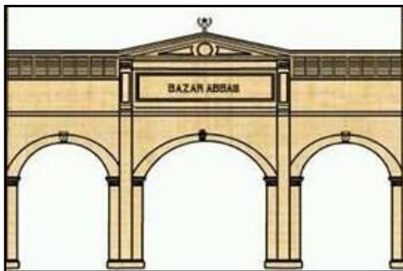
شكل رقم (٦) قطاع رأسى يوضح تفاصيل المدخل بالقسم الأوسط من الواجهة الرئيسية الجنوبية الشرقية للبازار - عمل الباحث
