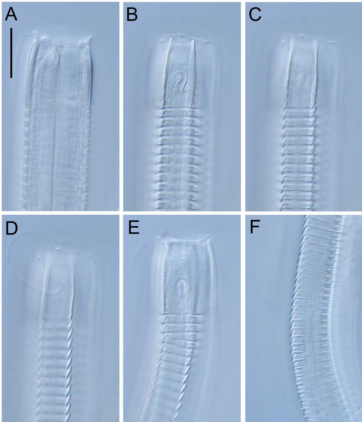
Fig. 8. Metadasynemoides taihua sp. nov., paratype, ♂ (NIWA 154948), light micrograph. A–E. Anterior body region. F. mid-body cuticle. Scale bar = 20 \mu m.
