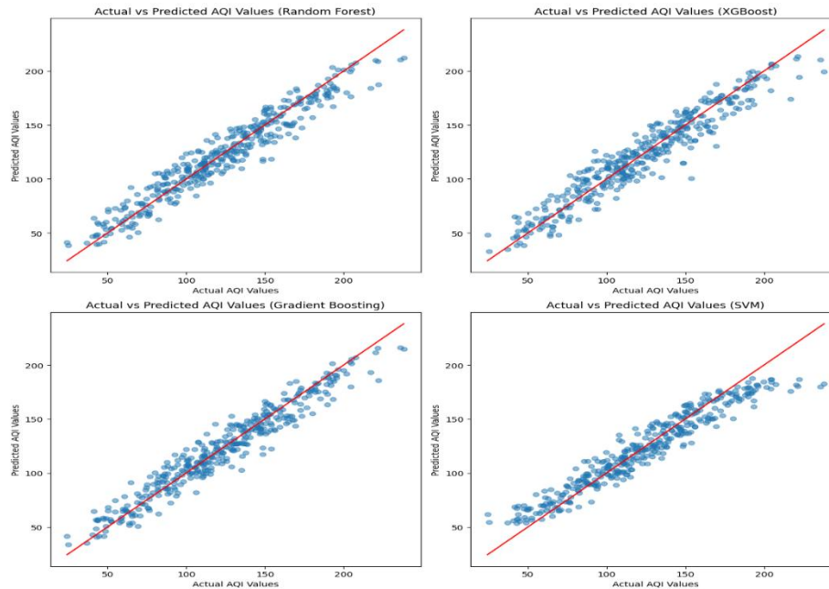
Figure 7. Actual vs Predicted AQI Values
