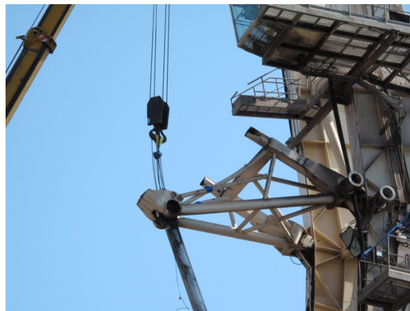
Figura 1: Zona di rottura del traliccio costituente il braccio della gru.
