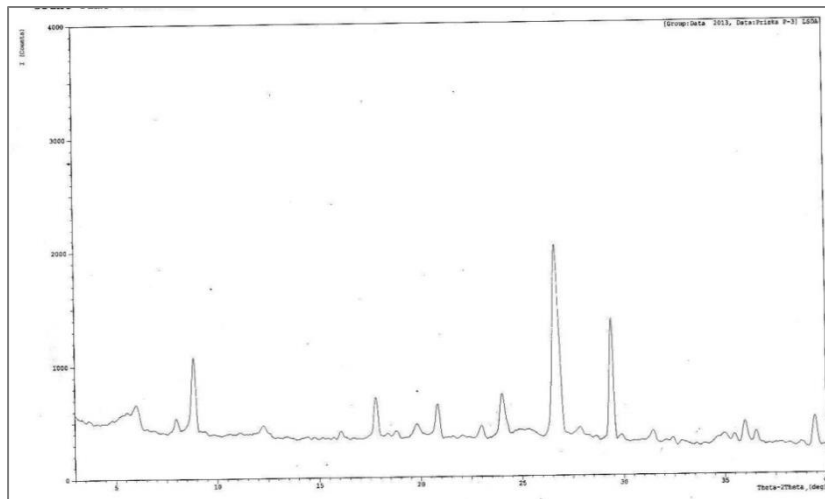
Gambar 2. Difraktogram lempung sebelum diaktivasi
