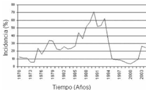
Figura 1. Comportamiento en Urabá, Colombia de la enfermedad de moko a través del tiempo según el número de fincas afectadas.
