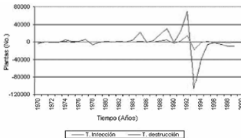
Figura 5. Tasas de infección y de destrucción de la enfermedad de moko en Urabá, Colombia.
