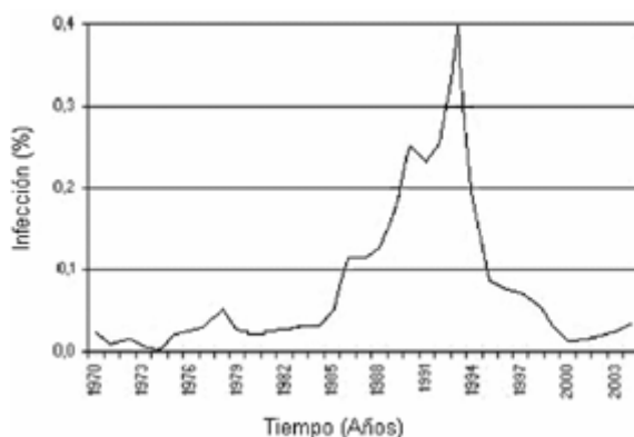
Figura 3. Dinámica de la infección por focos de la enfermedad de moko a través del tiempo en la zona de Urabá, Colombia.
