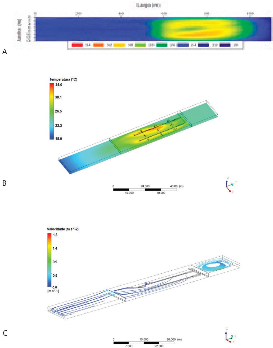
Figura 4. Condición nocturna primera semana de vida de las aves. Mapa de temperatura media a la altura de los pollitos a partir de los datos experimentales (A); mapa de temperatura media a la altura de los pollitos a partir del modelo en CFD (B) y mapa de turbulencia a partir del modelo en CFD (C).
