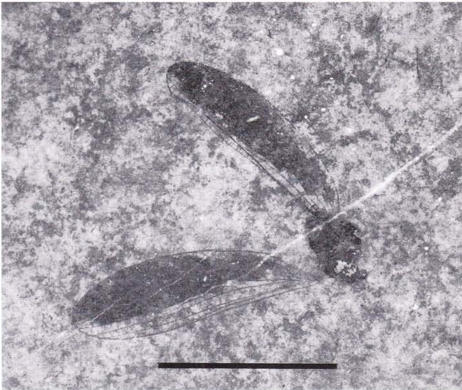
Fig. 5 - Wings of Tintorina meridensis n. sp. (MCSN 5001). Scale bar: 1 cm.
